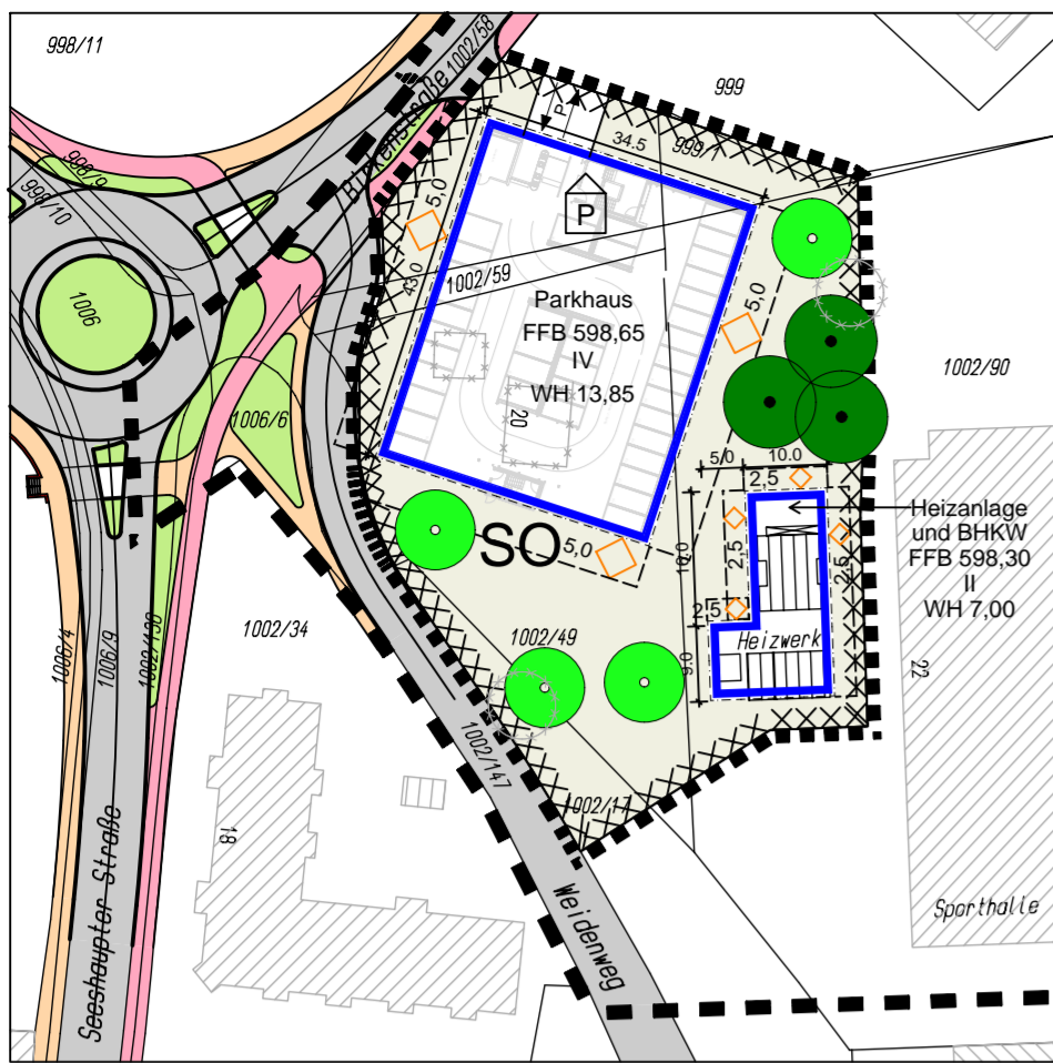
Lageplan M 1 : 1000
