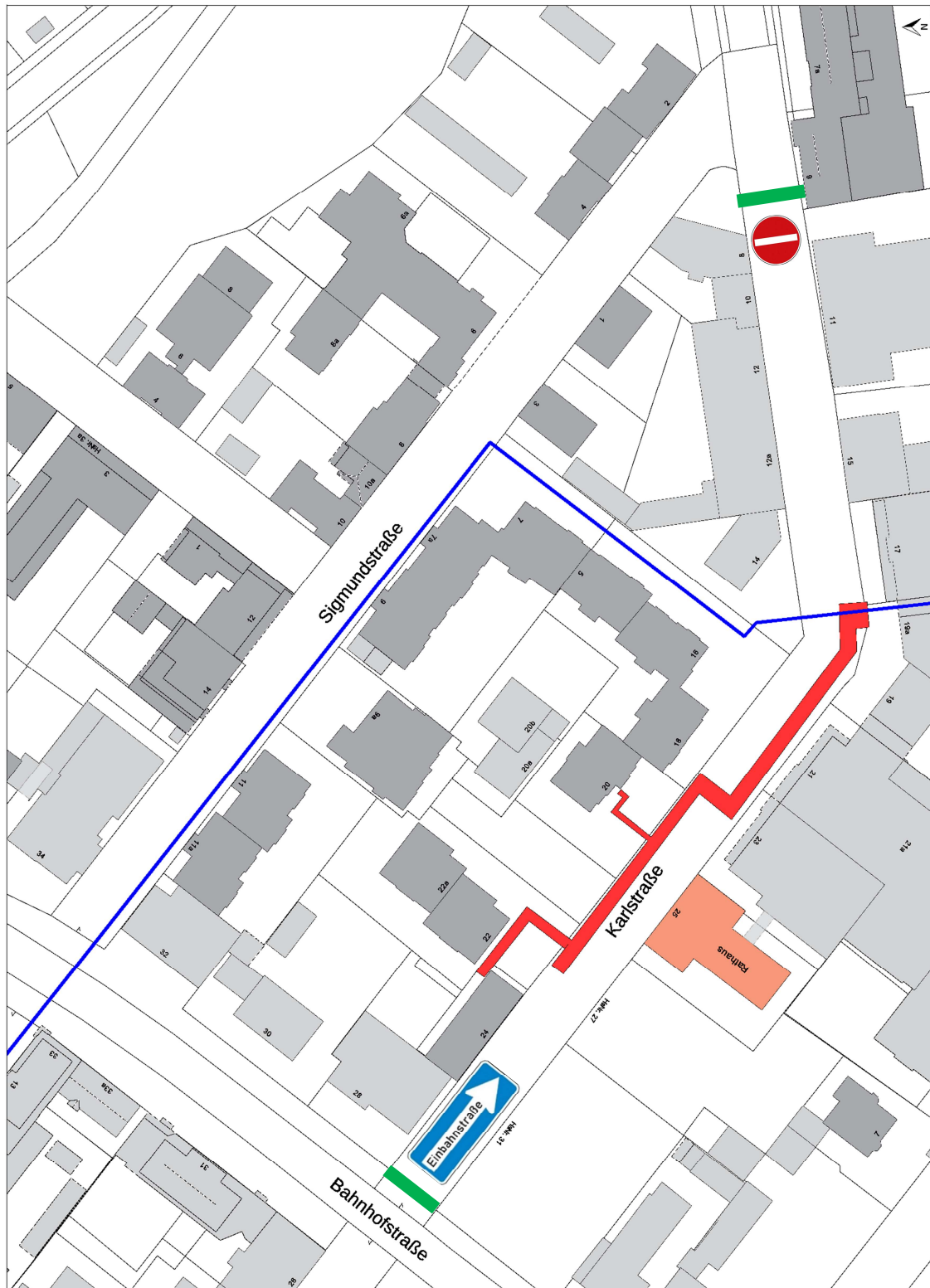
Übersichtsplan des Baubereichs (rot) in der Karlstraße, blaue Linie: bestehende Fernwärmetrasse, grüne Balken: Abschnitt mit Einbahnstraßenregelung
